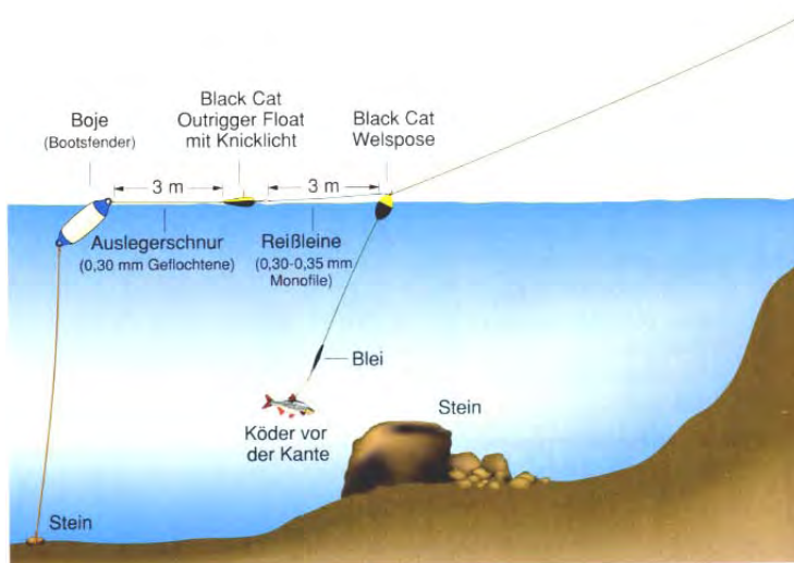
So sieht eine perfekt ausgebrachte Bojenmontage im Querschnitt aus.
